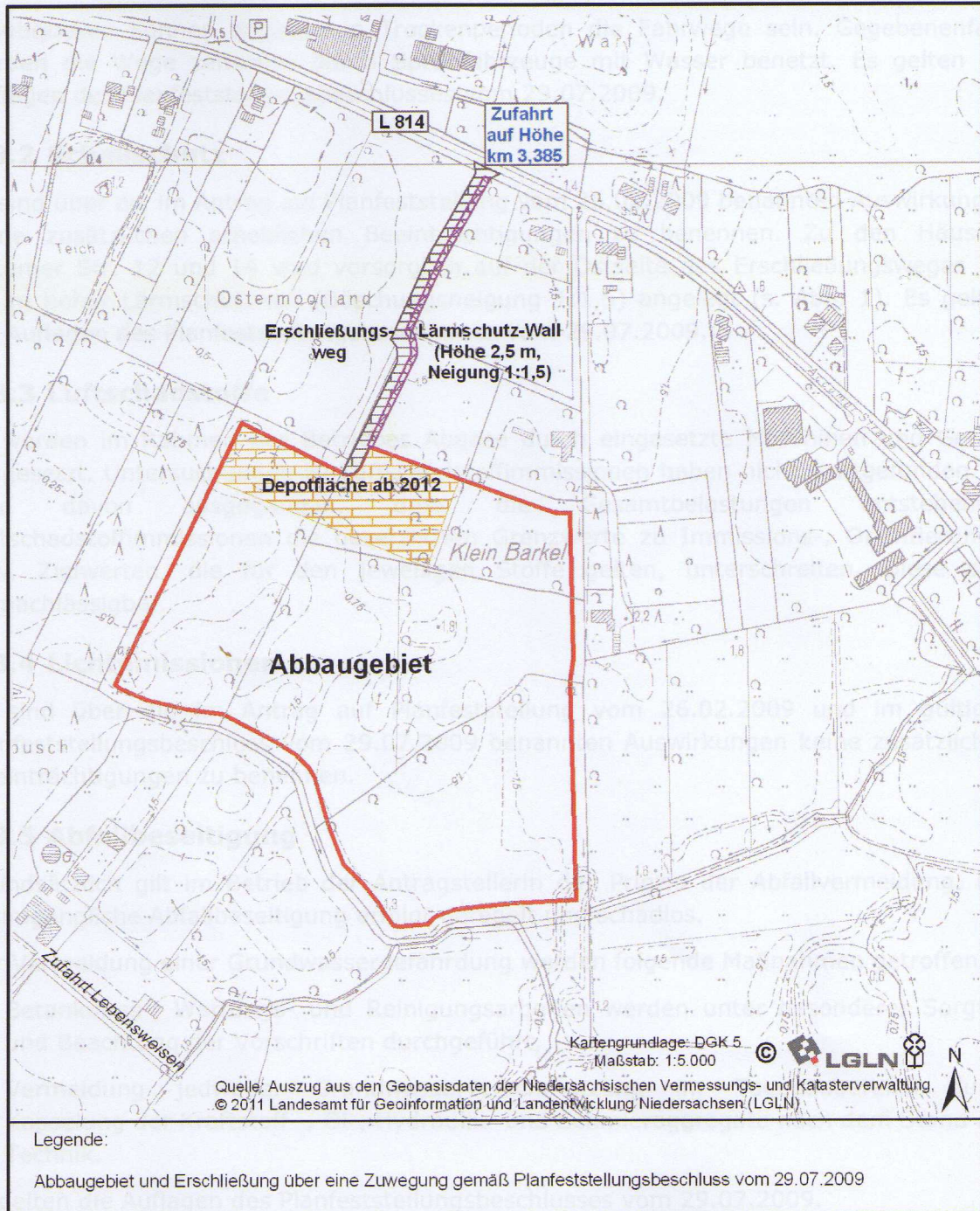
Abbildung 1: Geplante Zufahrt und Depotfläche ab 2012 im planfestgestellten Abbaubereich
